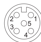
Schema del connettore Connector layout
